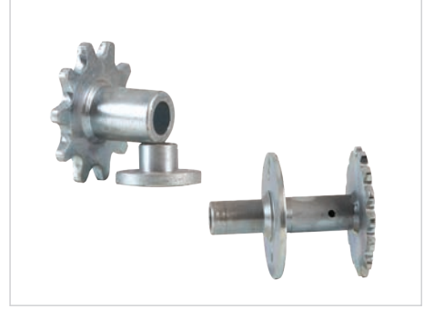
1048 Platin Serisi Gübrelı/Gübresız Çapa & Kültivatör Makara ve Dişliler (adet)
