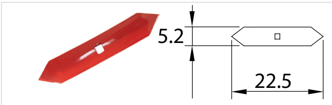
K-226 Birleşim Yaykürüm (Aysan) Bıçakları 7 mm (Yilandili)
