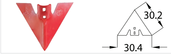
1114 BirleşimBOR 8 mm - 30 cm Kültivatör Bıçağı
