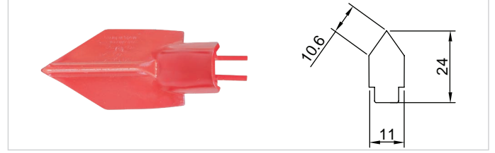
1102 Birleşim PlatinBOR 7 mm Çizel Pulluk Bıçağı
