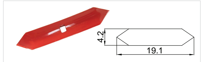
K-226 Birleşim Yayırcüm (Aysan) Bıçakları 7 mm (Yıldandılı)
