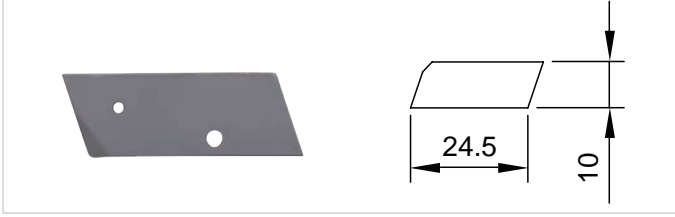
T-118 Alpler - Aydın 8 No Taban Demiri - Kısa
