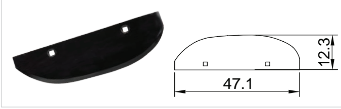
K-255 Pancar Söküm Bıçağı HARMAK
