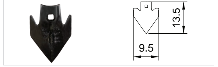
K-251 Birleşim-Aysan-Döşemen-BKS-Doğsan Kırlangıç Bıçak (Tekcivata) 9 cm
