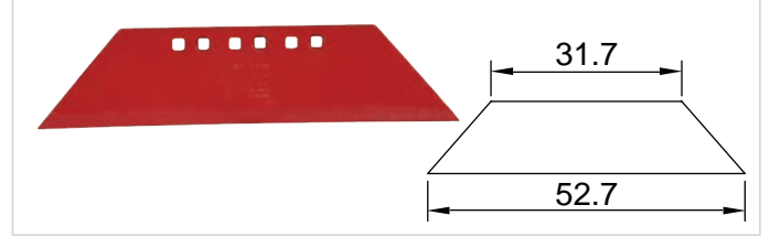
B-122 Turan 14 inç - 6 Delik
