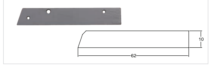
T-119 Alpler - Aydın 8 No Taban Demiri - Uzun
