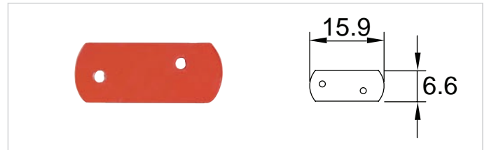
T-129 Ünlü Taban Demiri İç Parçası
