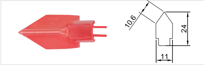
1103 Birleşim PlatinBOR 8 mm Çizel Pulluk Bıçağı
